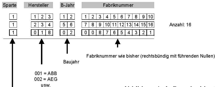
Abbildung 1: Aufbau der Identifikationsnummer
