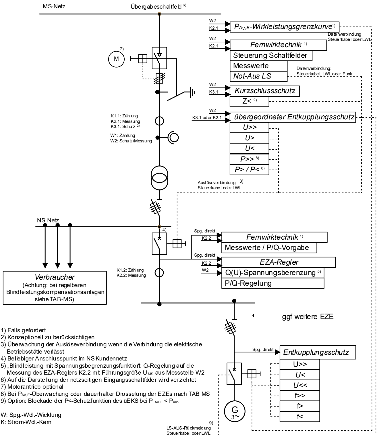
Bild D.11 Mischanlage – Beispiel für eine an das Mittelspannungsnetz angeschlossenen Kundenanlage mit Bezug und Erzeugungsanlage mit Lasttrennschalter und einer Erzeugungseinheit ohne Inselbetriebsmöglichkeit (Anschluss nicht in UW bzw. Schaltstation)
